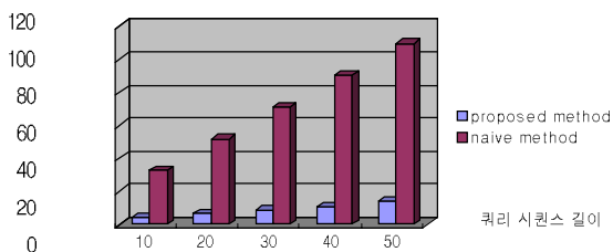
(그림 8) 질의 시퀀스의 평균 길이의 변화에 따른 평균 질의 처리 시간( k = 5, m = 500, \overline{L} = 200 )
