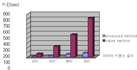
(그림 7) 데이터 시퀀스의 평균 길이 변화에 따른 평균 질의 처리 시간( k = 5, m = 500, |q| = 20 )
