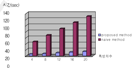
(그림 5) 특성 차수의 변화에 따른 평균 질의 처리 시간 ( m = 500 , \overline{L} = 200 , |q| = 20 )
